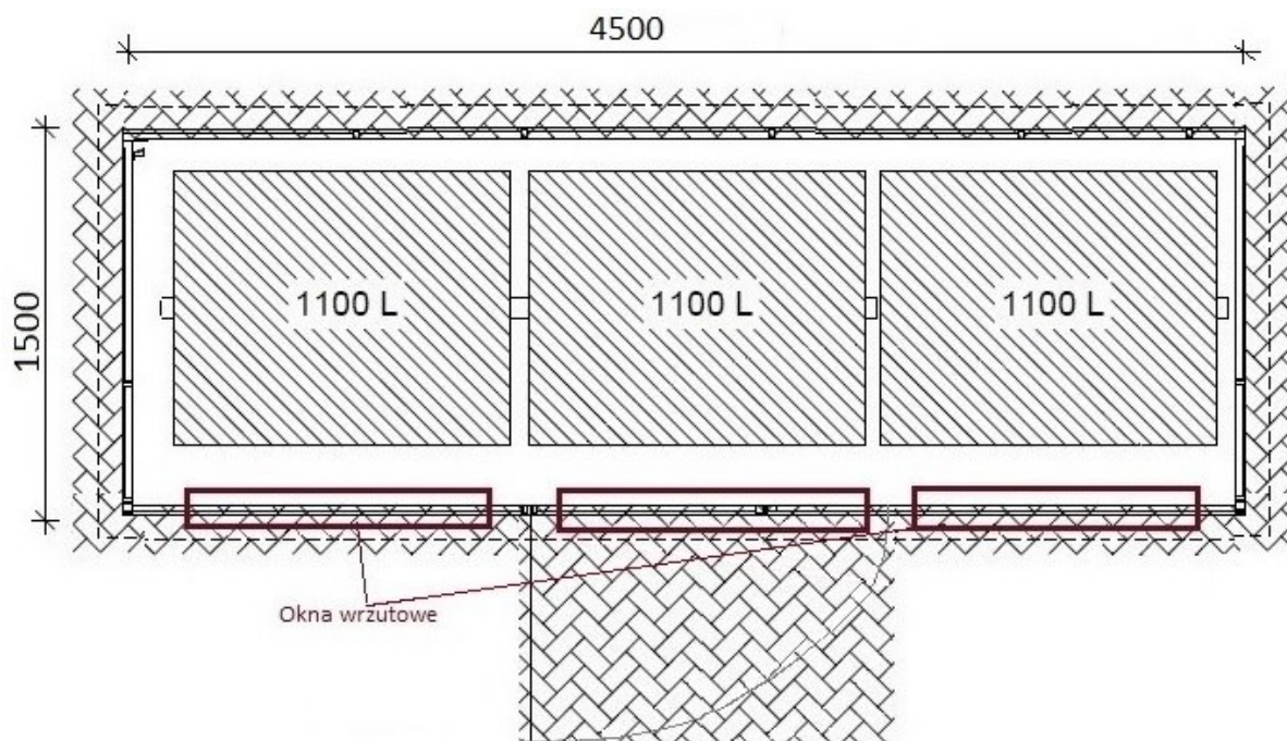
poglądowy rysunek techniczny rzut poziomy
