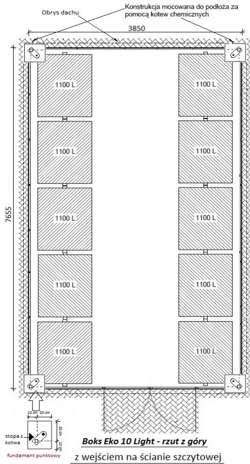
poglądowy rysunek techniczny rzut poziomy
