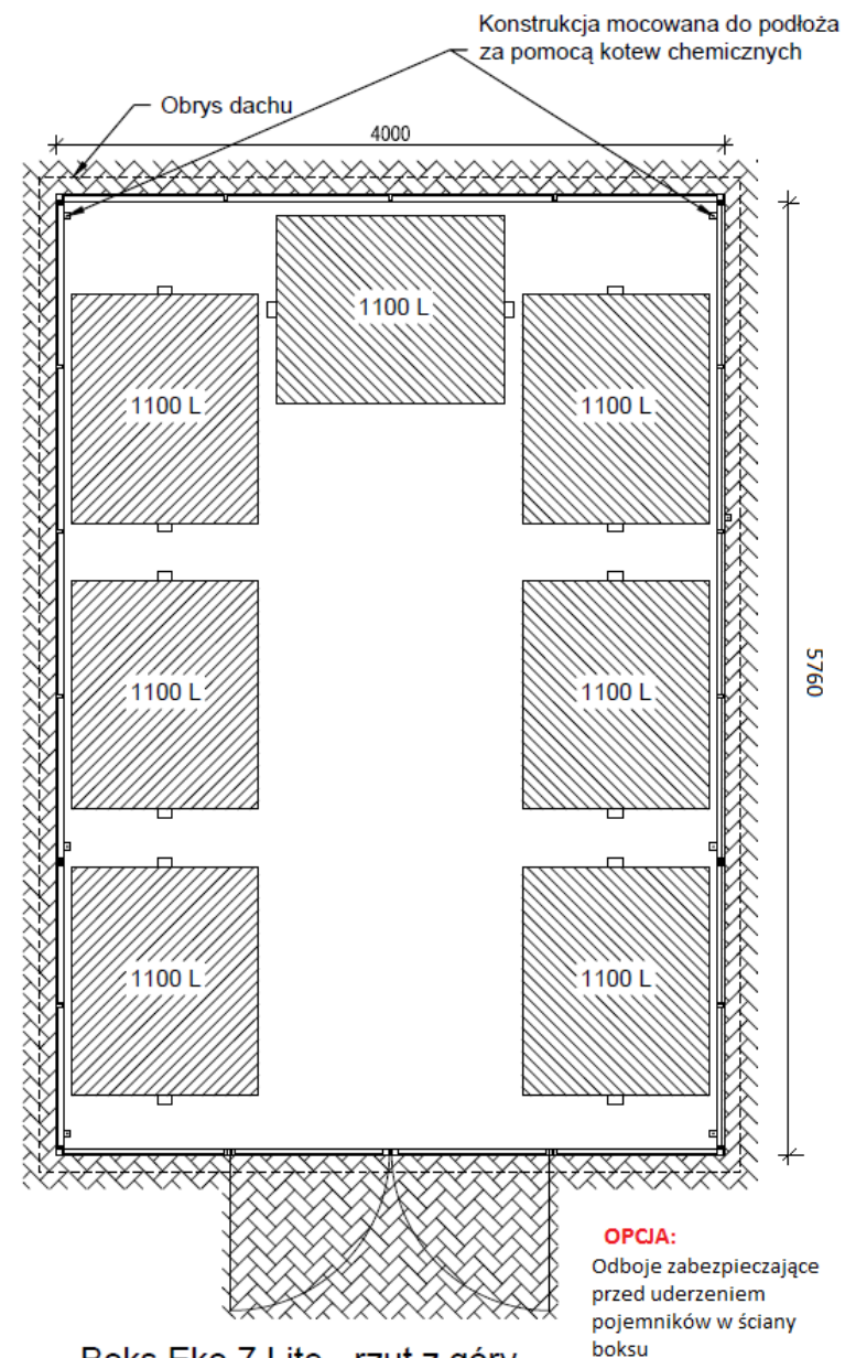
Boks Eko 7 Lite - rzut z góry z wejściem na ścianie szczytowej
