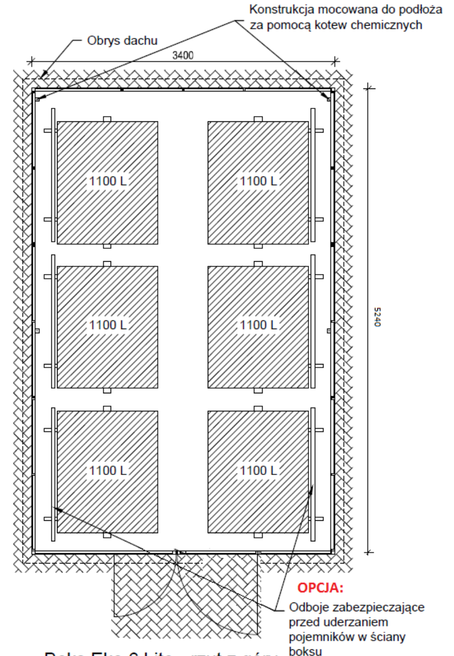
Boks Eko 6 Lite - rzut z góry z wejściem na ścianie szczytowej
