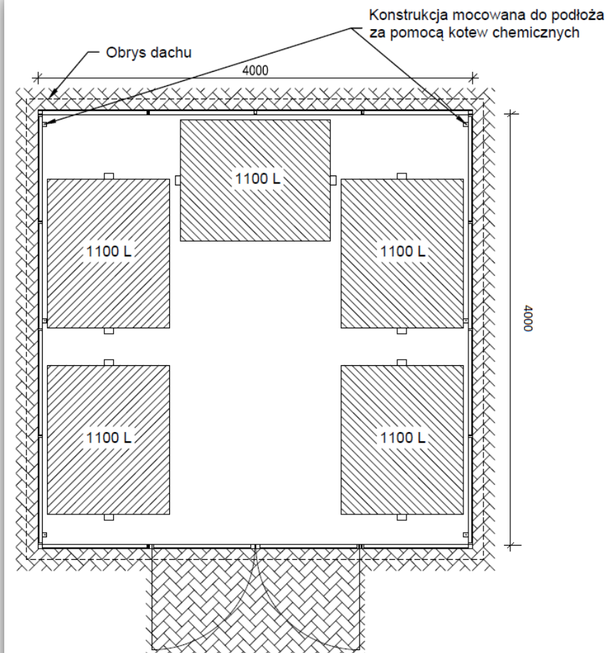
Boks Eko 5 Lite - rzut z góry z wejściem na ścianie szczytowej
