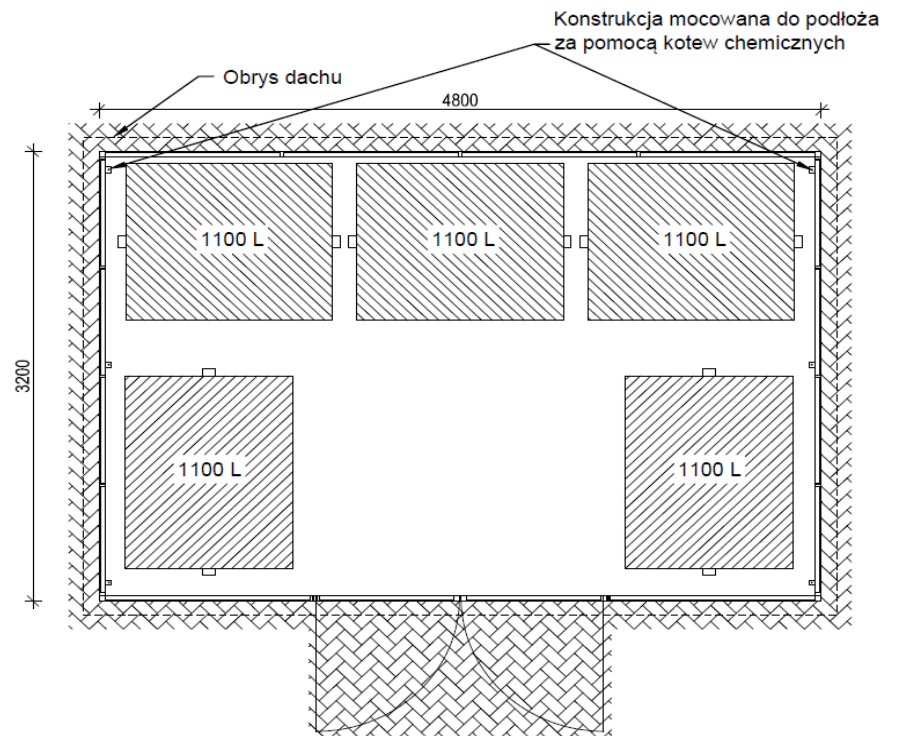
Boks Eko 5 Lite - rzut z góry
