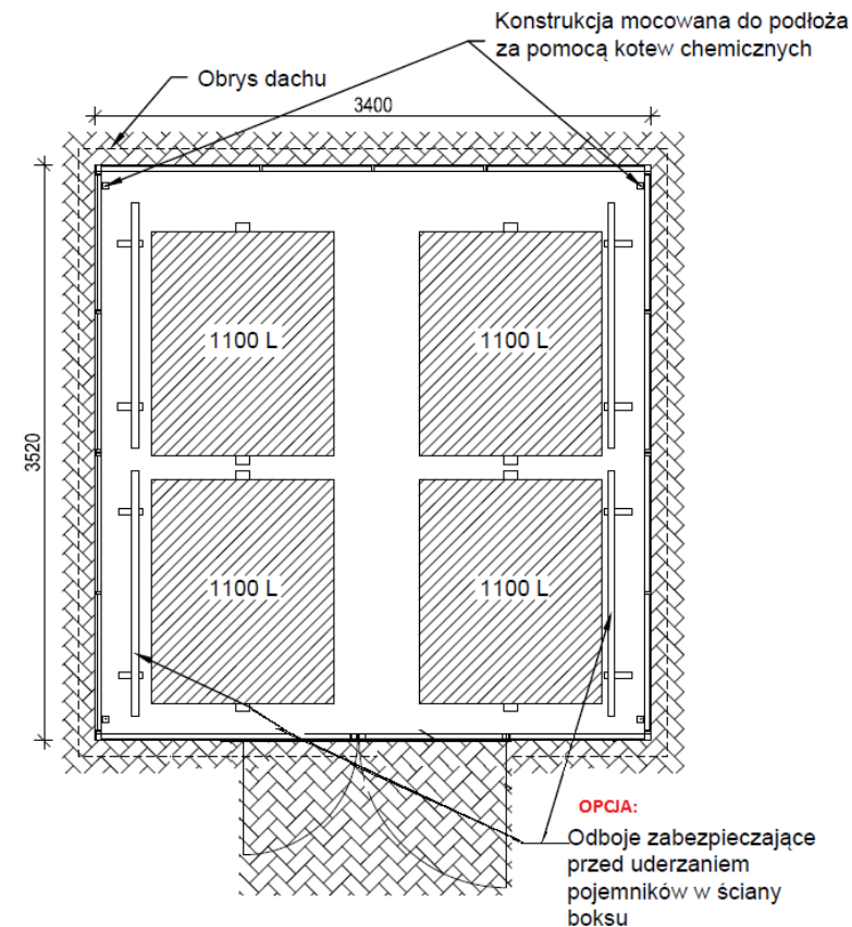
Boks Eko 4 Lite - rzut z góry z wejściem na ścianie szczytowej
