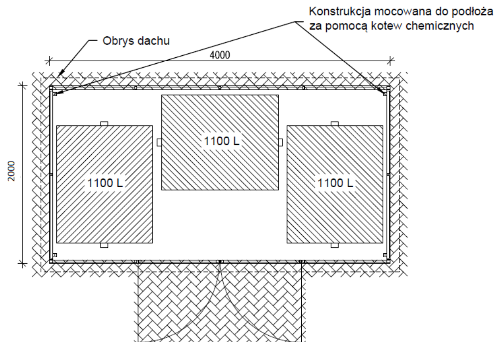
Boks Eko 3 - rzut z góry z wejściem na ścianie szczytowej
