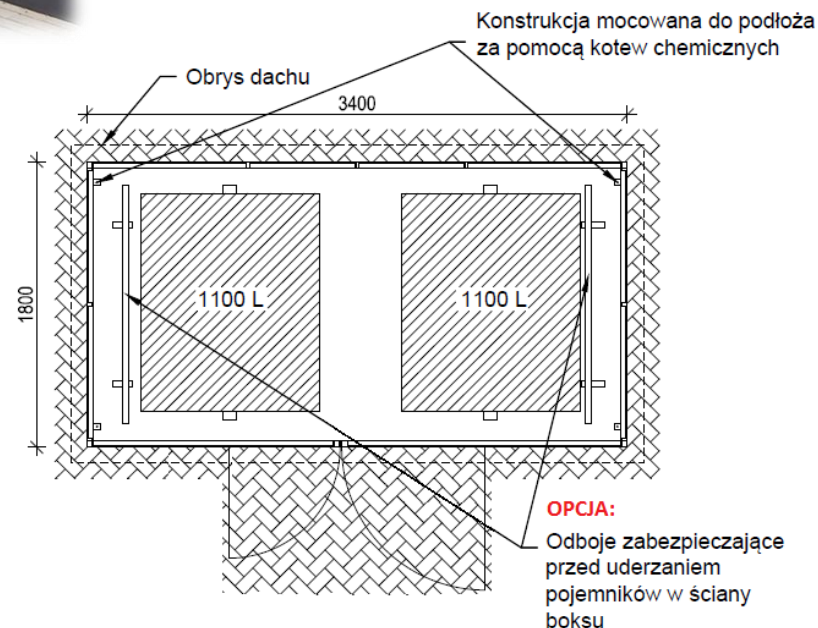
Boks Eko 2 Lite - rzut z góry
