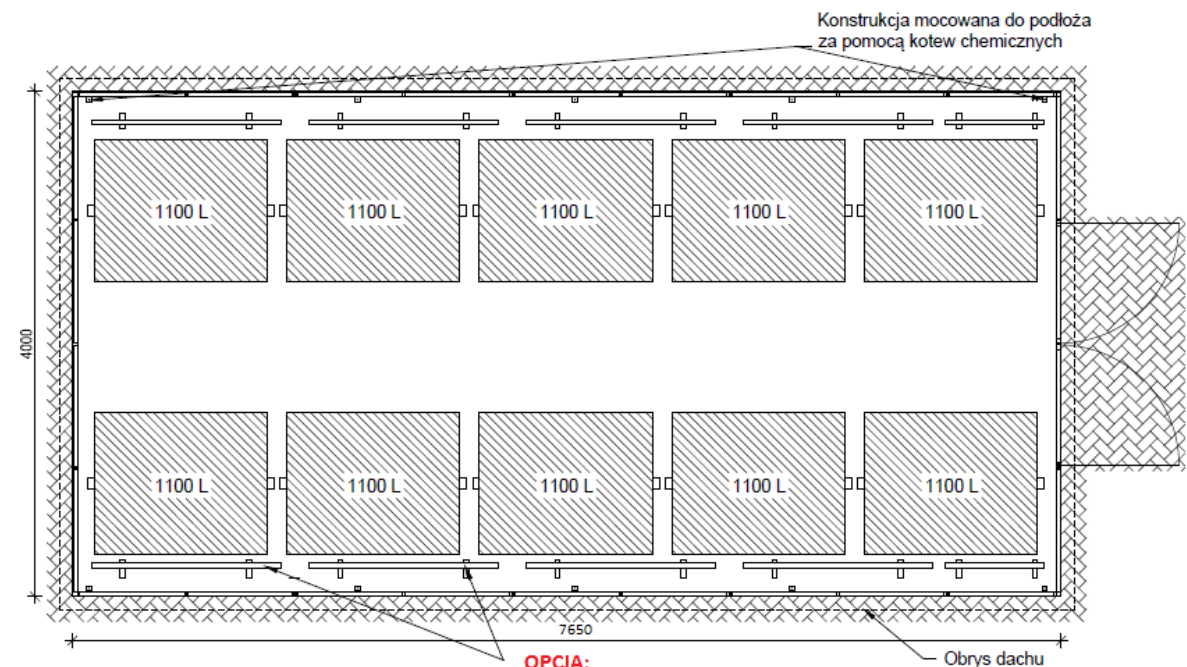
Boks Eko 10 Lite - rzut z góry z wejściem na ścianie szczytowej
