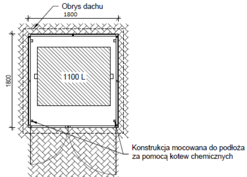
Boks Eko 1 Lite - rzut z góry
